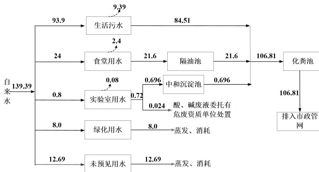
图 5.2-1 项目水平衡图 (单位: t/a)
