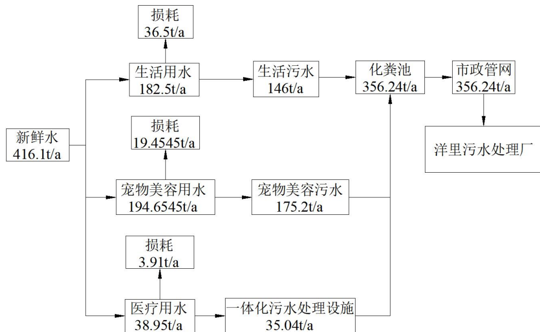
图 2.1-1 项目水平衡图
