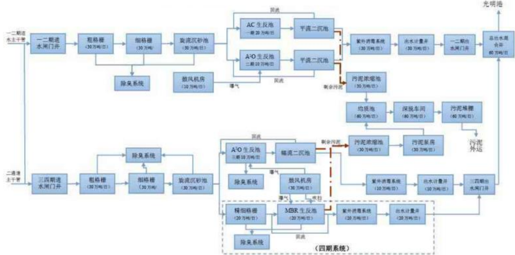
图 4.2-1 污水处理厂处理工艺流程图
