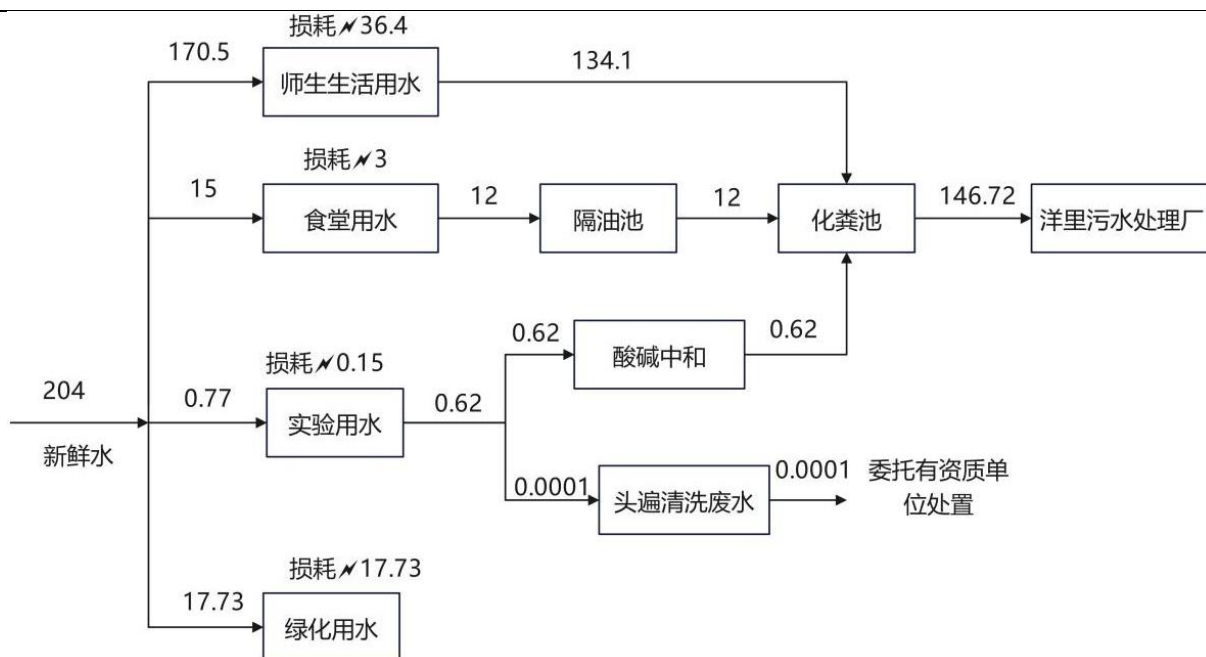
图2.2-1 项目水平衡图 (t/d)
